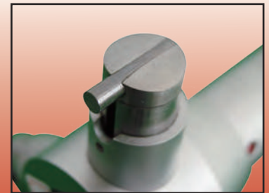
Blind hole type tungsten carbide anvil
