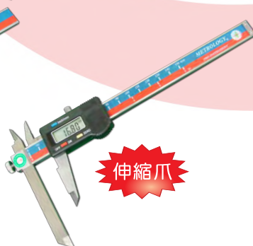
内外アンビル 換え可能
