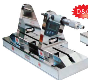
デジタルダイヤルゲージ校正器
