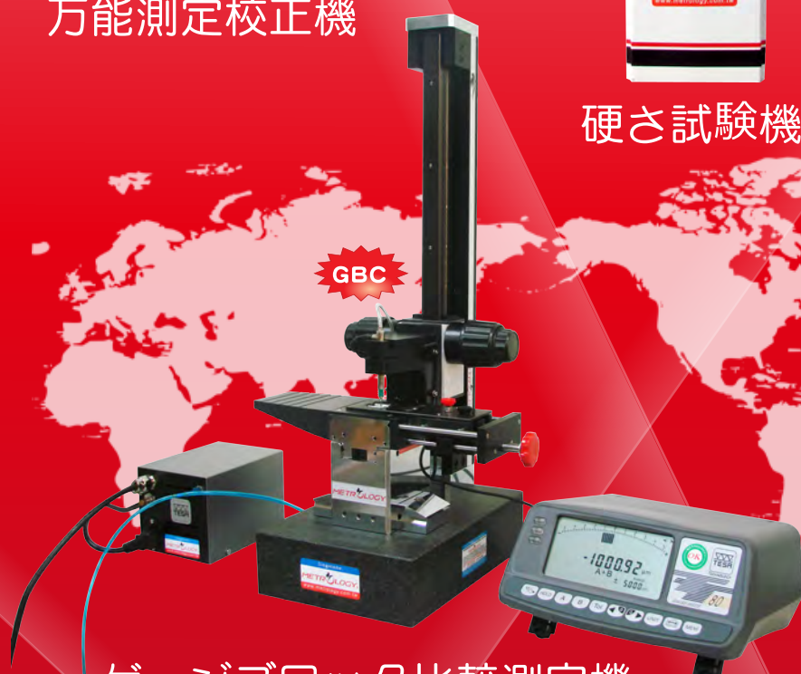
ゲージブロック比較測定機
