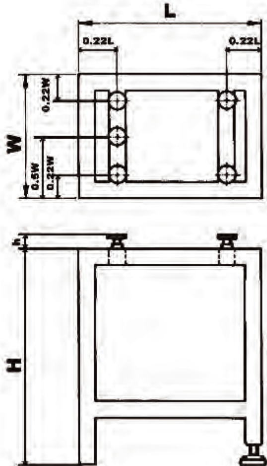
【腳架製作尺寸參考圖】
